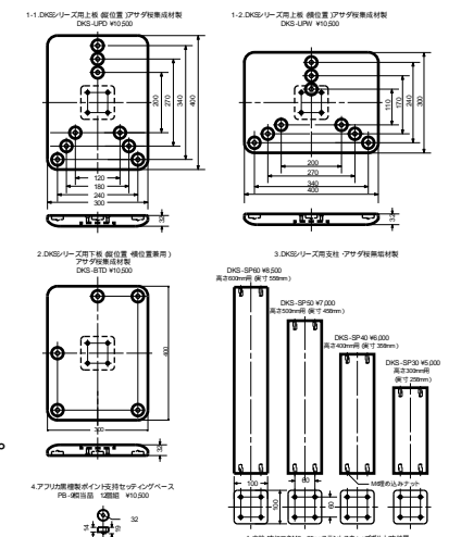
スピーカースタンドキットDKSシリーズシステムパーツ寸法図 細目単位はmm DKS-UPD 2枚、DKS-BTD 2枚、DKS-SP50 2本、PB-9 3個組み合わせた状態で W500x400mm (参考)
